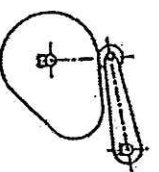
(d) Cam pair
